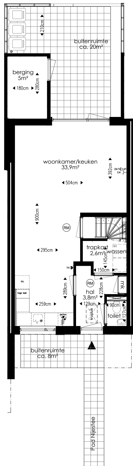
Begane grond
